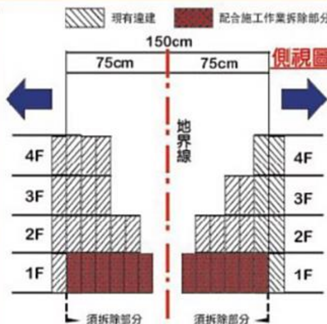
立面圖
